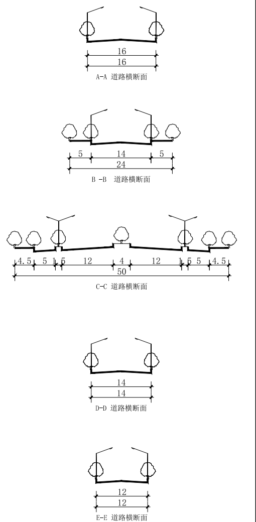
道路断面图
