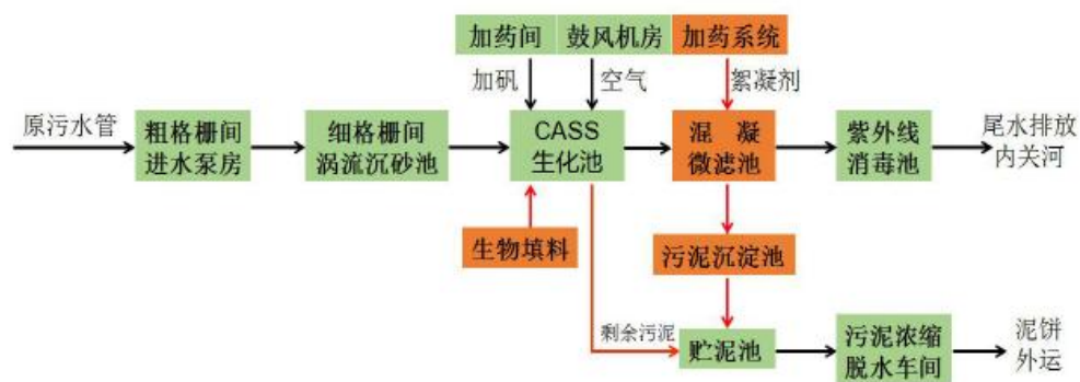
图4-3. 潮安区污水处理厂处理工艺
