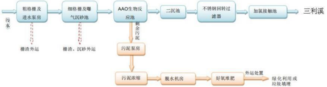
图 4-2 潮州市第二污水处理厂工艺流程图
