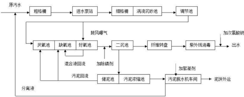
图4-3. 沙溪镇污水处理厂污水处理工艺流程图
